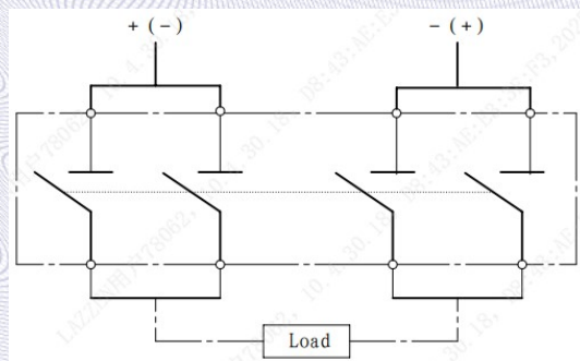
隔离器: DC1500V 接线图 2
