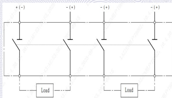
隔离器: DC1500V 接线图 3
